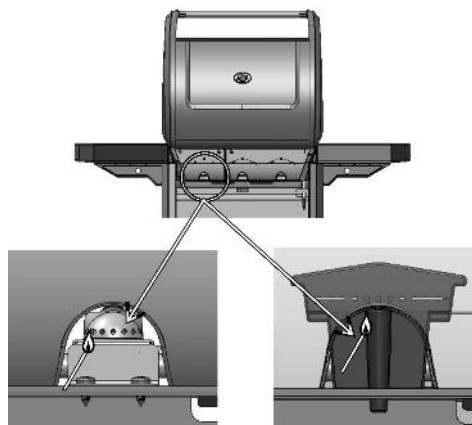
Brûleur acier
