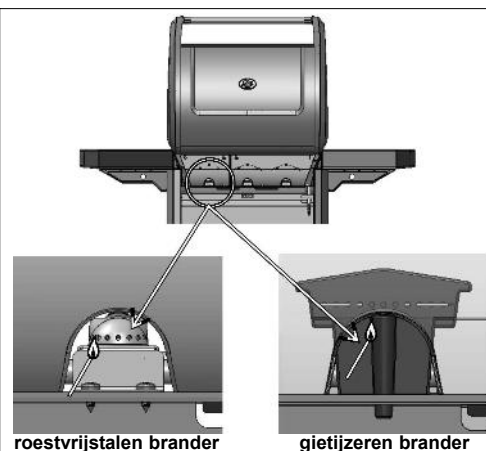
roestvrijstalen brander
