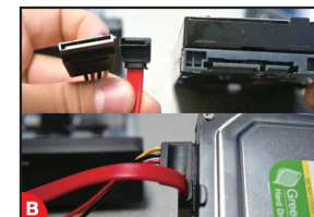
B Připojte SATA napájecí i datový kabel k disku HDD.
