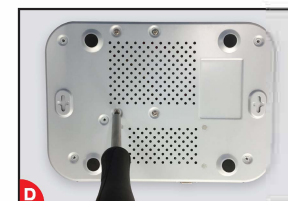
D Pomocí šroubků uchyťte disk HDD ze spodní strany rekordéru. Nasuňte horní kryt a upevněte šroubky.
