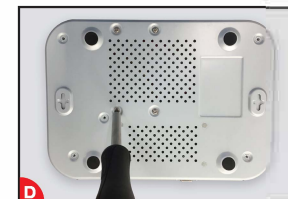
Trzymając dysk twardego i NVR, delikatnie go obróć, wyrównaj otwory na dysku twardym z otworami na NVR. Używając śrubokrętu Phillips, przykręć dostarczone wkretami. Załóż pokrywę.
