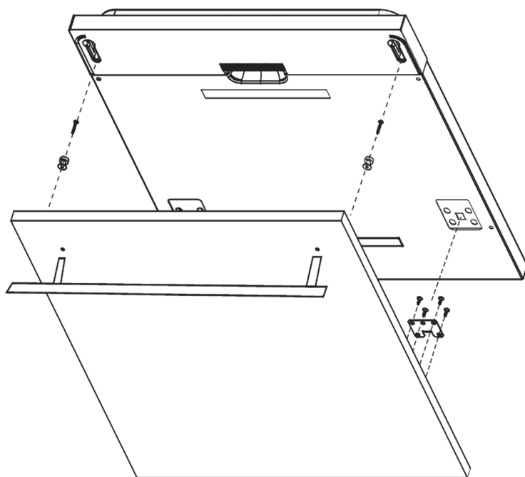
Obrázok 4a Inštalácia krycieho panelu
