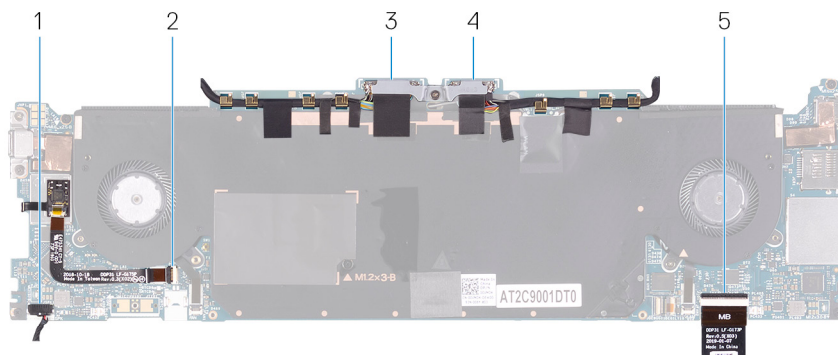
Obrázek 2. Konektory na základní desce
