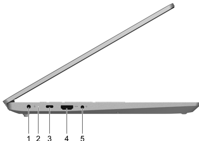
Obrázek 6. IdeaPad 5 (15", 05) a IdeaPad Slim 5 (15", 05) - pohled z levé strany
