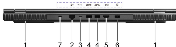
Obrázek 8. Pohled zezadu - 17" modely
