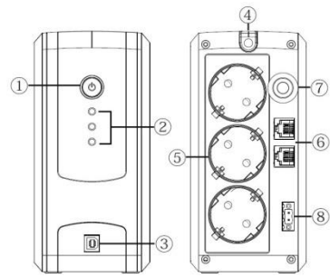
UT700EG (Schuko Outlet)
