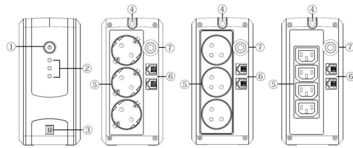
UT850EG / UT850EIG (Schuko/French/IEC Outlet)
